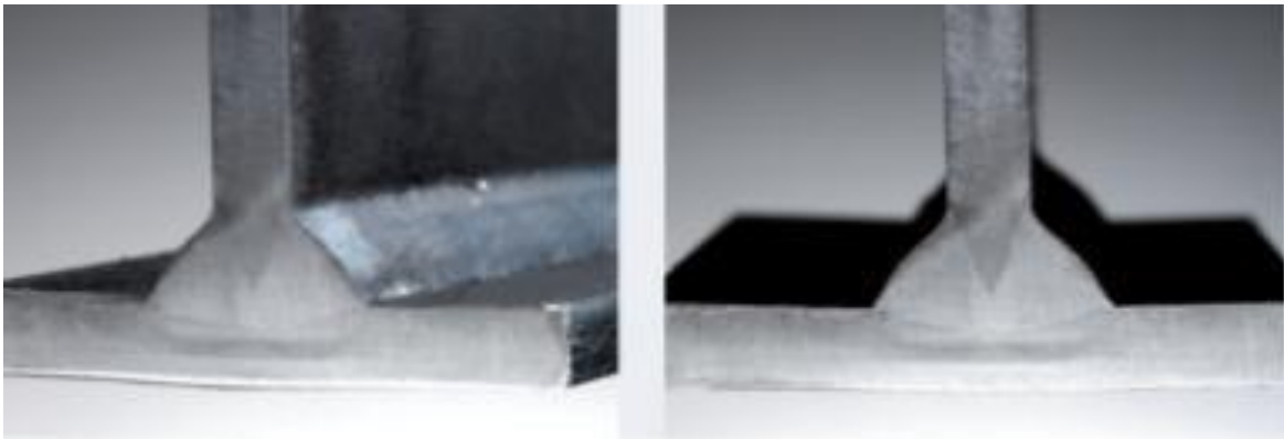
Slika 12. Prikaz kutnog spoja izvedenog RMT postupkom d=6 mm
