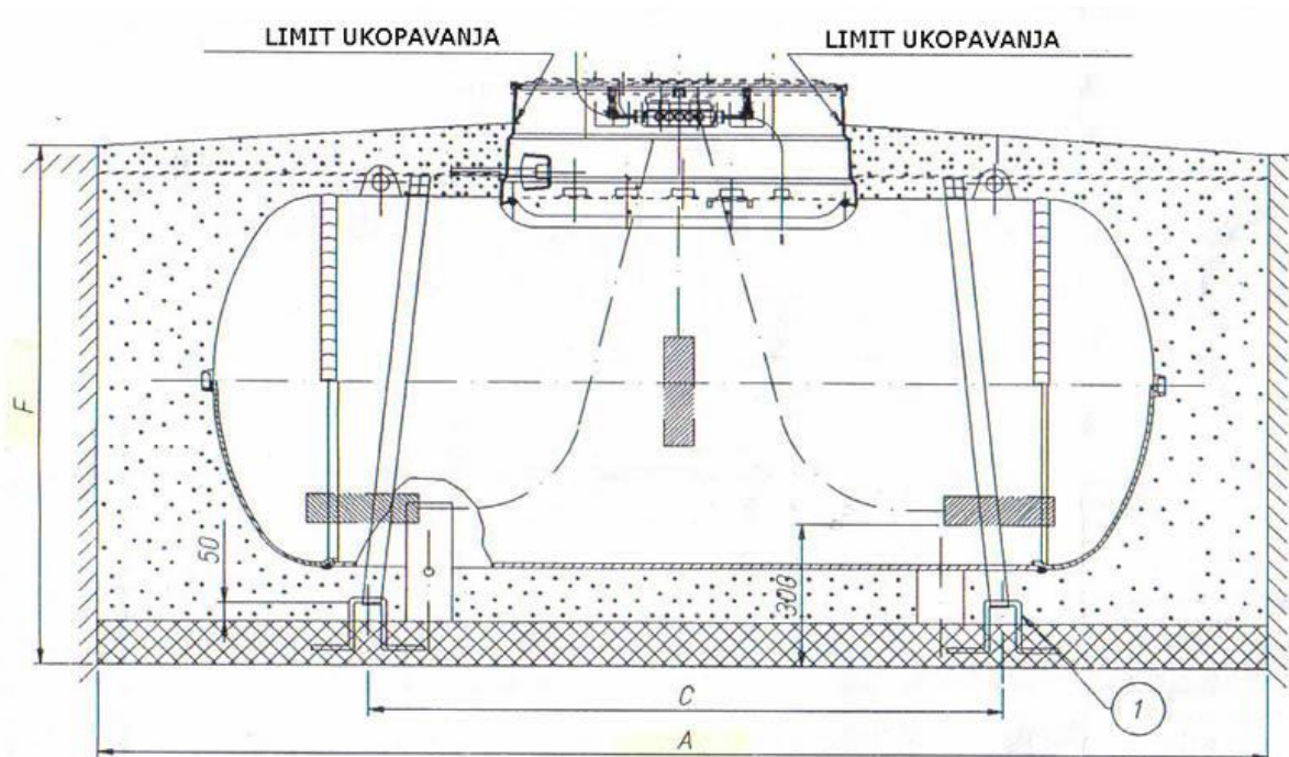
Slika 10. Podzemnog spremnika[10]
