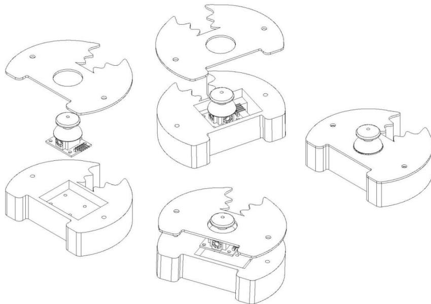
Slika 96. Kućište joysticka
