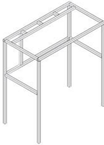
Slika 127. Konstrukcija postolja
