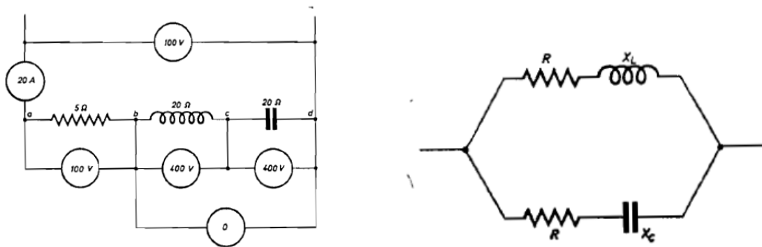
Slika 20. Serijski i paralelno spojeni elementi u rezonantnom krugu
