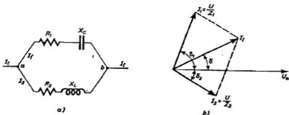
Slika 26. a) Paralelno spojeni elementi u krugu izmjenične struje; b) Odgovarajući vektorski dijagram
