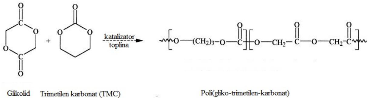
Slika 21. Dobivanje poli(gliko-trimetilen-karbonat) [39]
