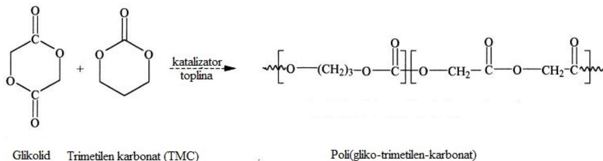
Slika 21. Dobivanje poli(gliko-trimetilen-karbonat) [39]
