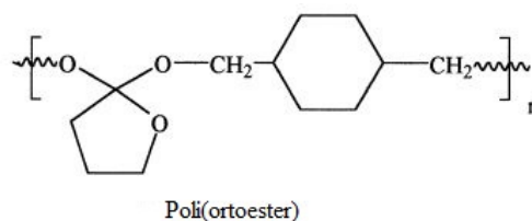
Slika 22. Struktura poli(ortoestera) [39]
