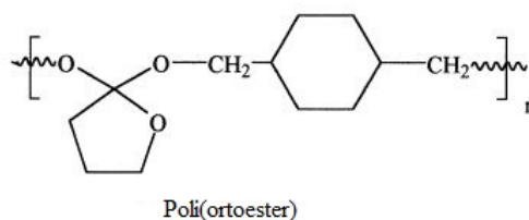
Slika 22. Struktura poli(ortoestera) [39]
