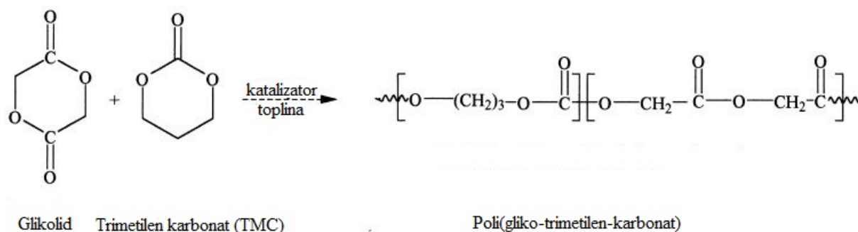
Slika 21. Dobivanje poli(gliko-trimetilen-karbonat) [39]
