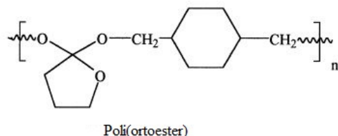
Slika 22. Struktura poli(ortoestera) [39]
