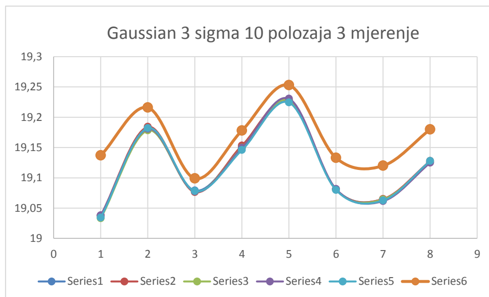
Slika 103. Gaussian 3 sigma za 10 položaja (3 mjerenje)
