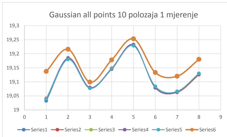
Slika 117. Gaussian all points za 10 položaja (1 mjerenje)
