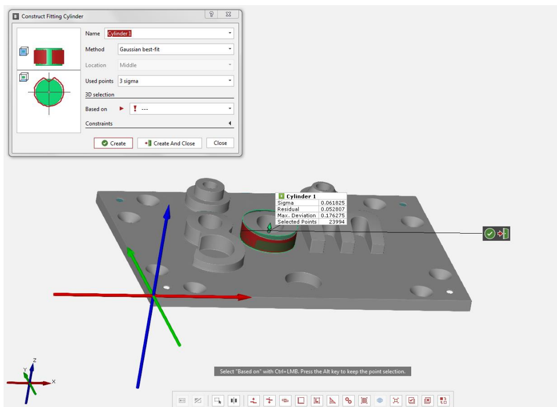
Slika 26. Odabir cilindra
