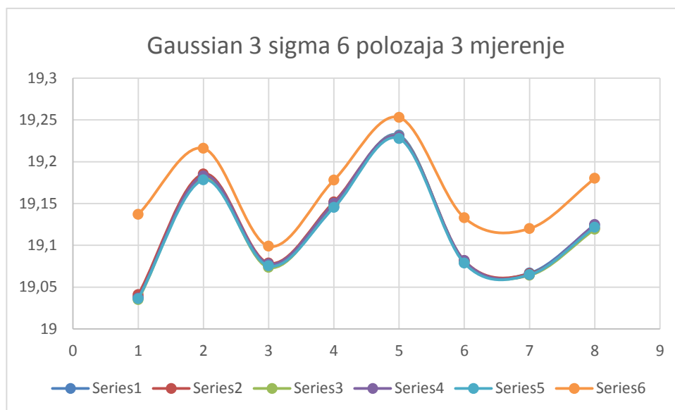
Slika 102. Gaussian 3 sigma za 6 položaja (3 mjerenje)
