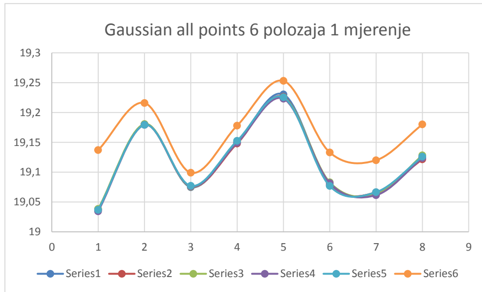
Slika 116. Gaussian all points za 6 položaja (1 mjerenje)
