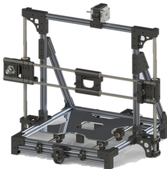
Slika 32. Openbeam printer [36].
