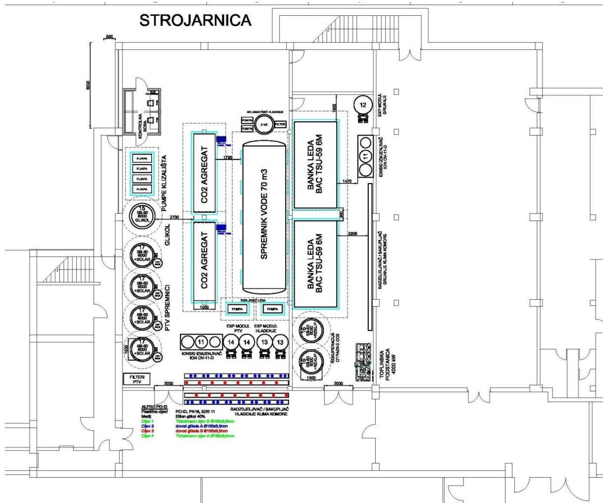
Slika 18: Strojarnica
