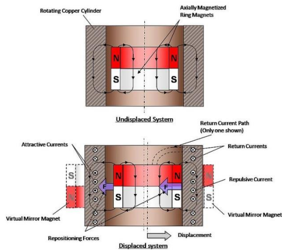
Slika 16. Magnetsko zrcalo
