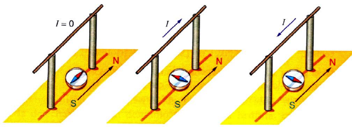
Slika 1. Oerstedov eksperiment
